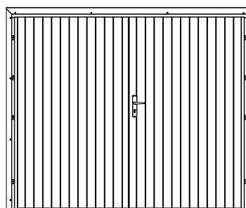
Nr. 46 Double door / Doppeltür 70 mm 2370 x 1955 mm - R -
