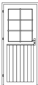
Nr. 41 Door / Einzeltür 40 mm / Standard+ 840 x 1955 mm - L
