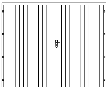
Nr. 40 Double door / Doppeltür 40 mm 2370 x 1955 mm - R
